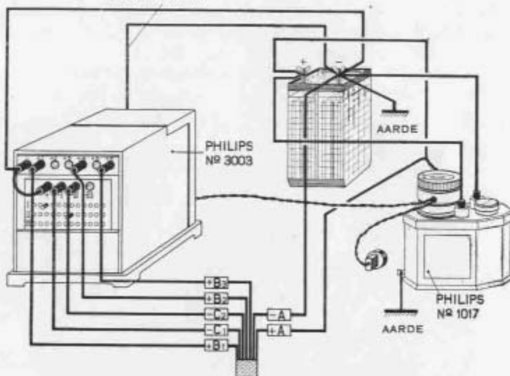
Fig. 3 Bij gebruik van Philips plaatspanningapparaat No. 3003 en Philips gelijkrichter No. 1017 (De neg. roosterspanning van bus -I is op -4 V, van bus -II op -15 V ingesteld)
